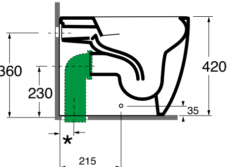
OCECVT/K Curva tecnica per foro a 60/70mm dalla parete. Technical bend for 60/70 mm hole from the wall.
