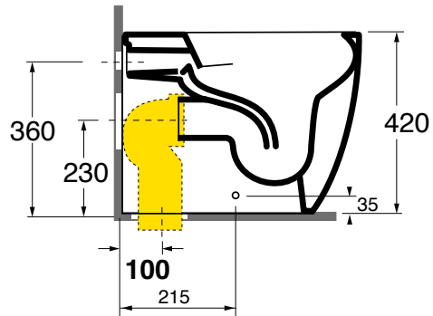
OCECVT Curva tecnica per foro a 100mm dalla parete. Technical bend for 100mm hole from the wall.
