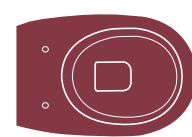
PVS Vaso sospeso Wall-hung wc 51,5 x 35,5 x h27
