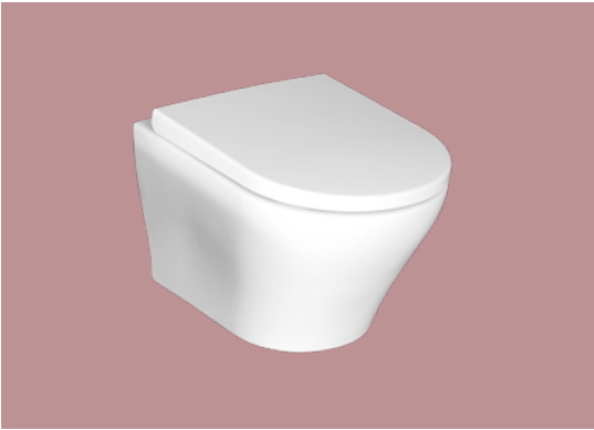
DVS - 50,5 x 36 x h31 23 kg
