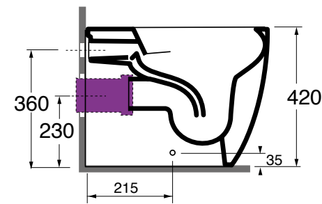
OCER Collettore per foro parete H230 mm. Technical bend for wall hole H230.
